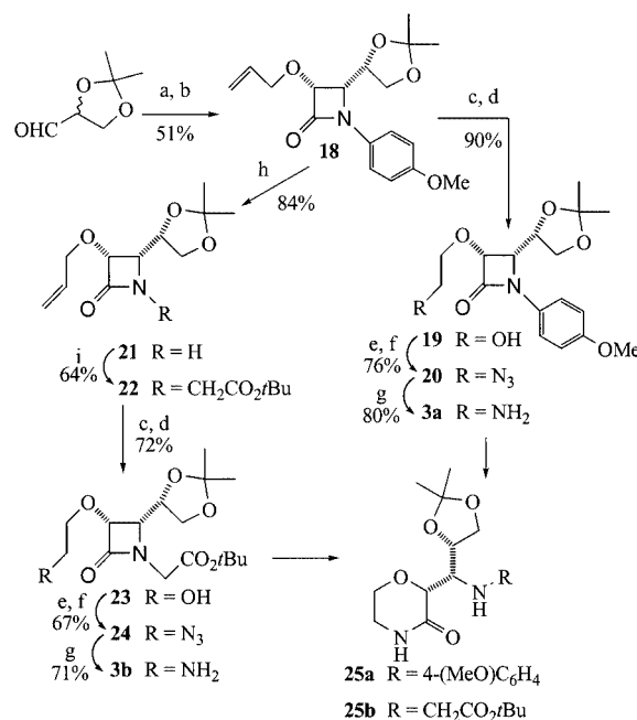
Scheme 4. a) p -Anisidine, mol. sieves; b) allyloxyacetyl chloride, \text{CH}_2\text{Cl}_2 , \text{Et}_3\text{N} , -20\text{ }^\circ\text{C} to room temp.; c) \text{O}_3 , \text{CH}_2\text{Cl}_2/\text{MeOH} , then \text{Me}_2\text{S} ; d) \text{BH}_3\cdot\text{THF} ; e) \text{MsCl} , \text{Et}_3\text{N} , \text{CH}_2\text{Cl}_2 , -30\text{ }^\circ\text{C} ; f) \text{NaN}_3 , \text{DMF} , 50\text{--}60\text{ }^\circ\text{C} ; g) \text{Ph}_3\text{P} , \text{H}_2\text{O}/\text{THF} , room temp.; h) \text{Ce}(\text{NH}_4)_2(\text{NO}_3)_6 ; i) t\text{BuOK} , \text{BrCH}_2\text{CO}_2t\text{Bu} , n\text{Bu}_4\text{NI}
