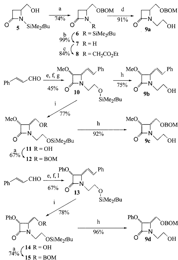
Scheme 2. a) BOMCl, Et 3 N; b) n Bu 4 NF, THF, −40 °C; c) KOH, BrCH 2 CO 2 Et; d) Ca(BH 4 ) 2 , THF/H 2 O, −20 °C; e) HOCH 2 CH 2 NH 2 ; f) Me 2 tBuSiCl, Et 3 N; g) MeOCH 2 COCl, Et 3 N, CH 2 Cl 2 , −78 °C → room temp.; h) HF, H 2 O/CH 3 CN; i) O 3 , then Me 2 S·NaBH 4 ; l) PhOCH 2 COCl, Et 3 N, CH 2 Cl 2 , −78 °C → room temp.
